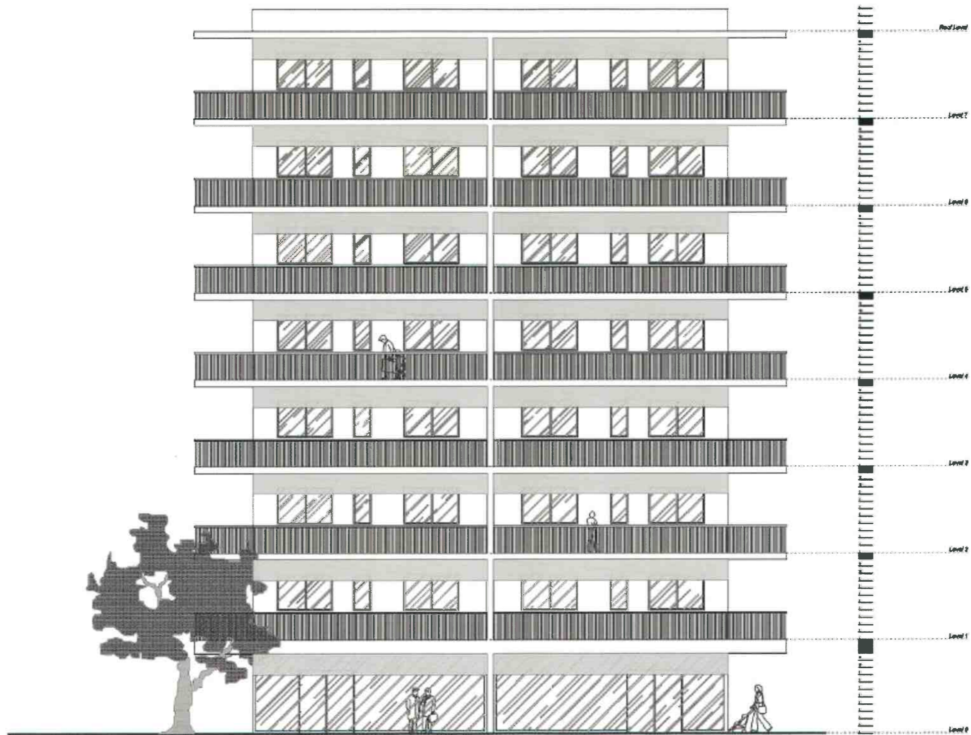
Elevation B Scale: 1:100
